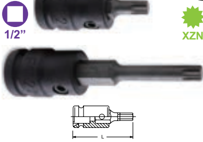
BUSSOLA MASCHIO ESAGONALE IN DUE PARTI: BUSSOLA + INSERTO MASCHIO XZN
