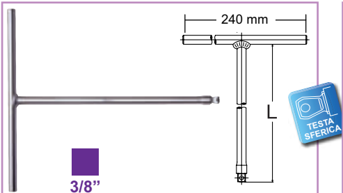
CHIAVI A "T" MASCHIO QUADRO 3/8" TESTA SFERICA CON IMPUGNATURA LARGHEZZA 240 MM
