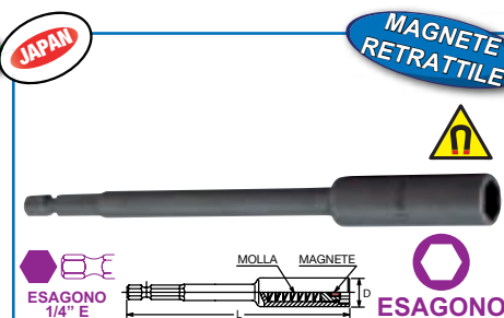
CON MAGNETE RETRATTILE SCARICO INTERNO 25 MM
