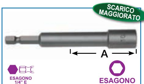
CHIAVI A BUSSOLA ESAGONALI AD ALTA RESISTENZA CON SCARICO MAGGIORATO ESECUZIONE INTEGRALE
