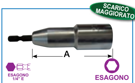
CHIAVI A BUSSOLA ESAGONALI ATT. 1/4" CON SCARICO INTERNO 60 MM
